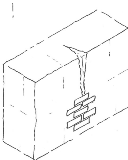
Figure 28: Reprise en adobes
