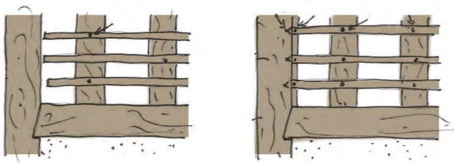
Fig 2: Exemple de liaison entre support et structure (croquis Franck Lahure)
