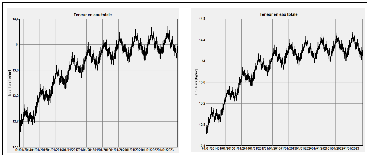
Figure 36 - Graphes d'évolution de la teneur en eau total de la paroi, isolation intérieure PSE, avec (droite) et sans (gauche) défaut d'étanchéité à l'air
