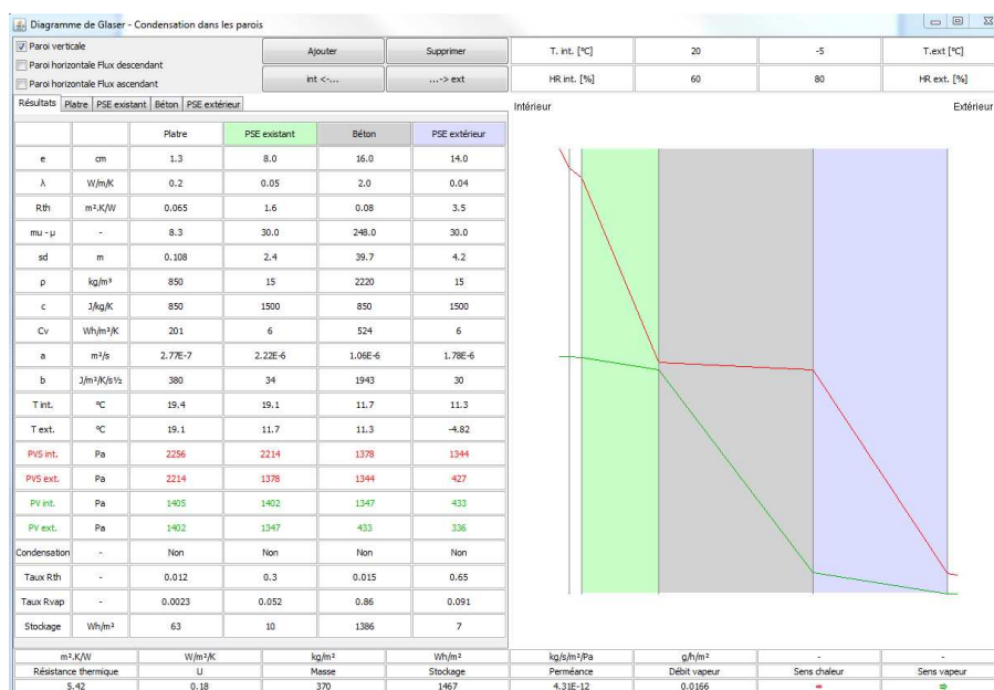
Figure 30 - Glaser : ITI + ITE réno, -5°C ext
