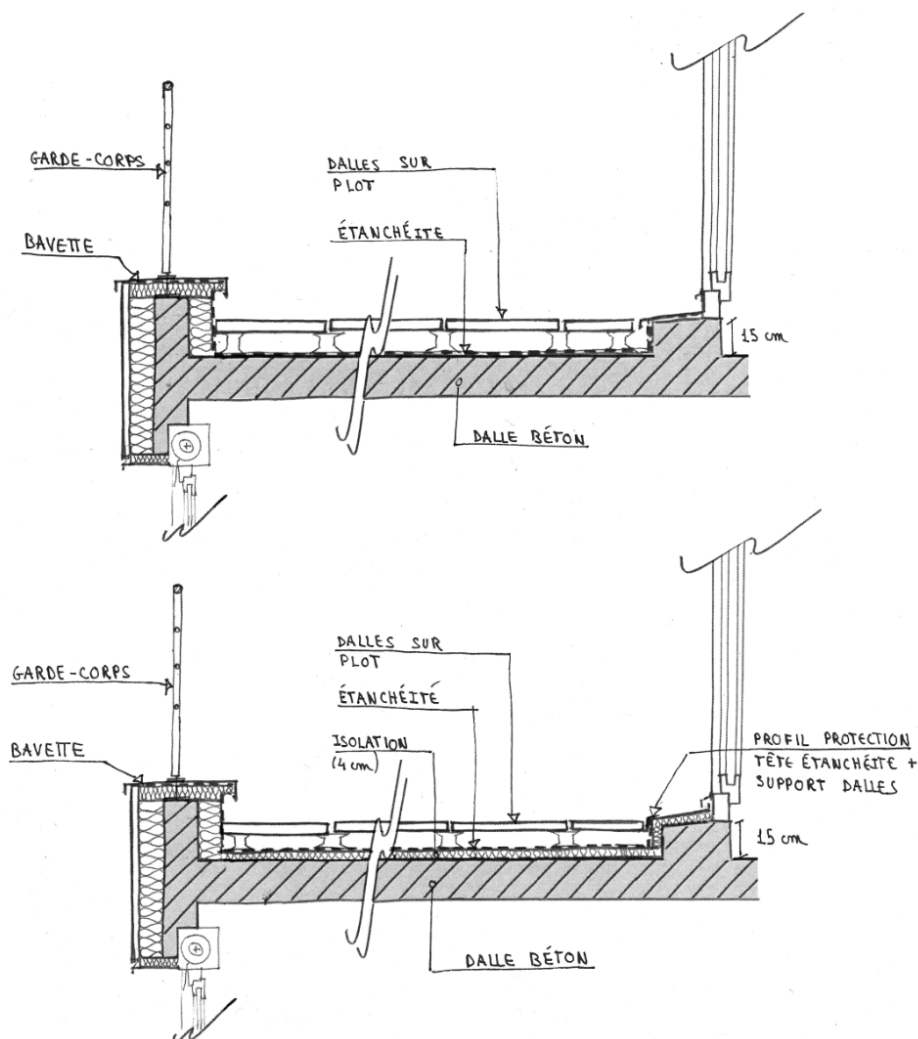
Figure 20 - Isolation d'un toit terrasse accessible par le logement en attique
